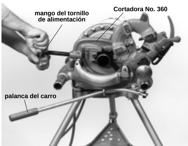
Figura 9 – Corte de tubos con la Cortadora No. 360
