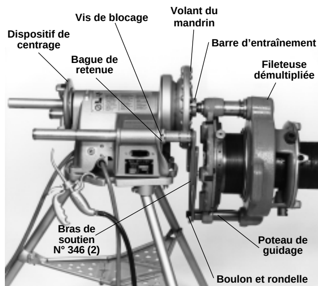
Figure 20 – Fileuse démultipliée en couplage direct avec le système d'entraînement
