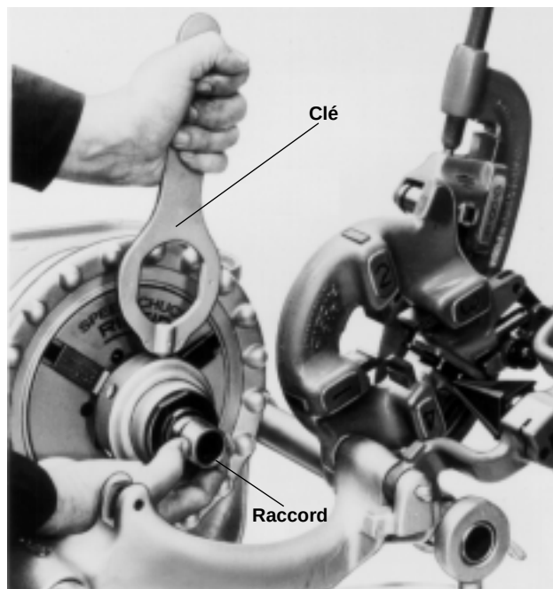
Figure 25 – Libération du raccord du mandrin à raccords
