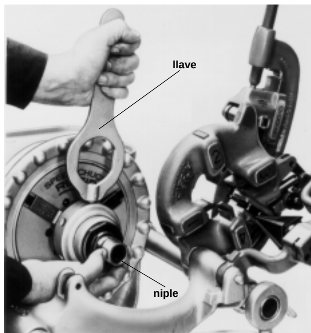
Figura 25 – Desenganche del niple del portaherramientas niplero
