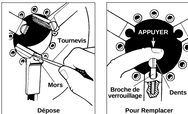
Figure 26 – Remplacement des mors
